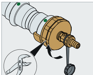
4. Hvis det ved påfyllingen av et anlegg oppstår en lekkasje, ettertrekk den avtrykbare pluggen med egnet verktøy. Viega anbefaler trykktesting med luft.
