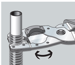
1. Kutt beskyttelsesrøret med saksen for beskyttelsesrør (modell 5341).
